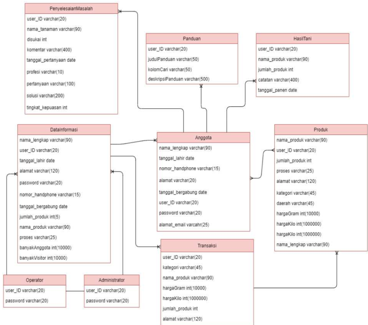
Gambar 2. Struktur sistem eduFarm
