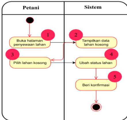
Gambar 3. Activity Diagram Penyewaan Lahan
