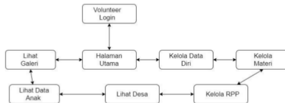
Gambar 4.5 Tampilan struktur navigasi volunteer.
