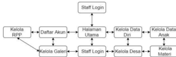
Gambar 4.4 Tampilan struktur Navigasi Staff.
