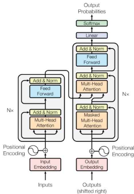
Gambar 2. Model arsitektur transformer [9]
