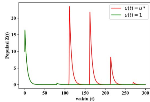
Gambar 6. Perbandingan solusi numerik populasi pemangsa jenis kedua Z(t)
