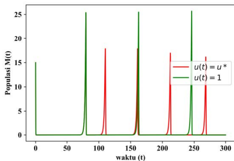
Gambar 5. Perbandingan solusi numerik populasi mangsa M(t)
