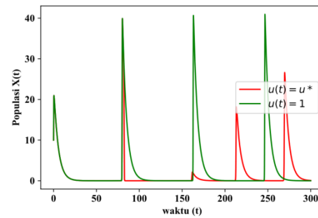
Gambar 3. Perbandingan solusi numerik populasi pemangsa jenis pertama yang sehat X(t)
