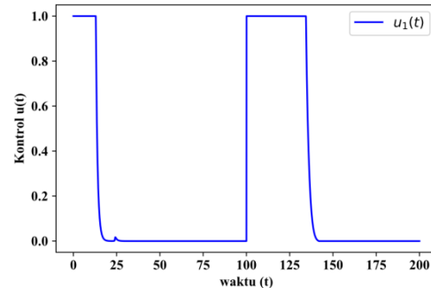
Gambar 9. Kontrol u_1(t) yang menyatakan pemberian vaksinasi pada t \in [0, 200]
