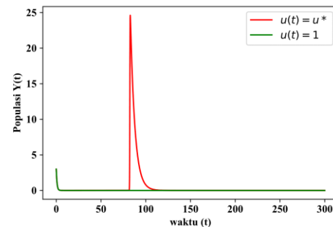
Gambar 4. Perbandingan solusi numerik populasi pemangsa jenis pertama terinfeksi Y(t)
