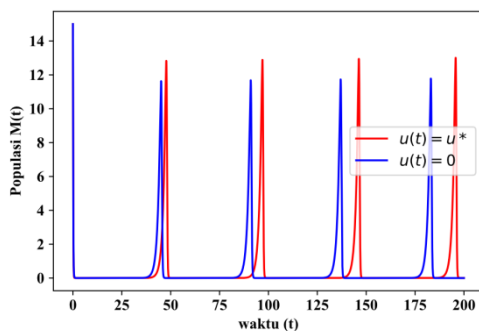
Gambar 8. Perbandingan solusi numerik populasi mangsa M(t) dengan kontrol persamaan (22) dan tanpa kontrol.
