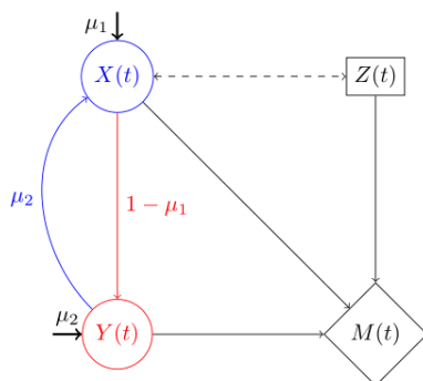
Gambar 2. Skema interaksi antara populasi mangsa dan pemangsa
