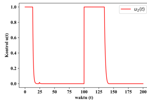
Gambar 10. Kontrol u_2(t) yang menyatakan pemberian treatment pada t \in [0, 200]
