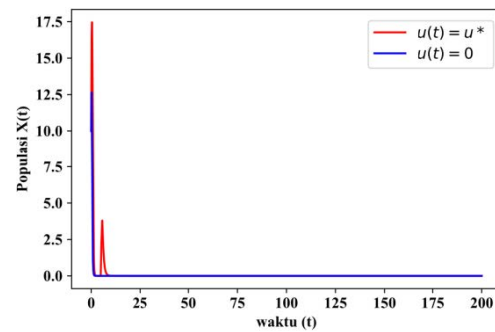
Gambar 7. Perbandingan solusi numerik populasi pemangsa jenis pertama X(t) dengan kontrol persamaan (22) dan tanpa kontrol
