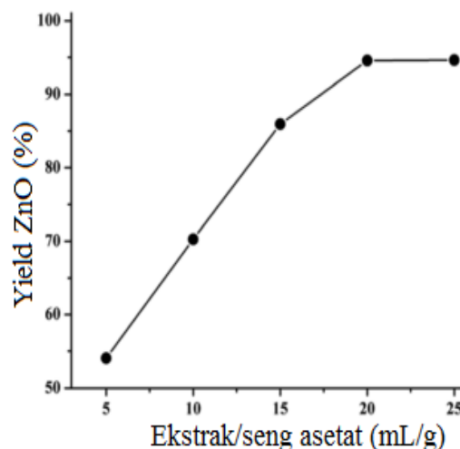
Gambar 11. Pengaruh kadar ekstrak tanaman terhadap yield ZnO
