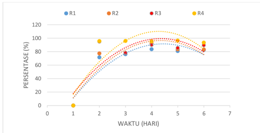
Gambar 2. Grafik Efisiensi Penurunan Fosfat
