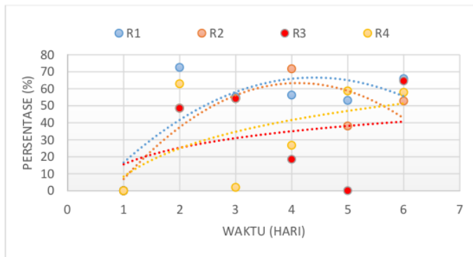
Gambar 1. Grafik Efisiensi Penurunan COD
