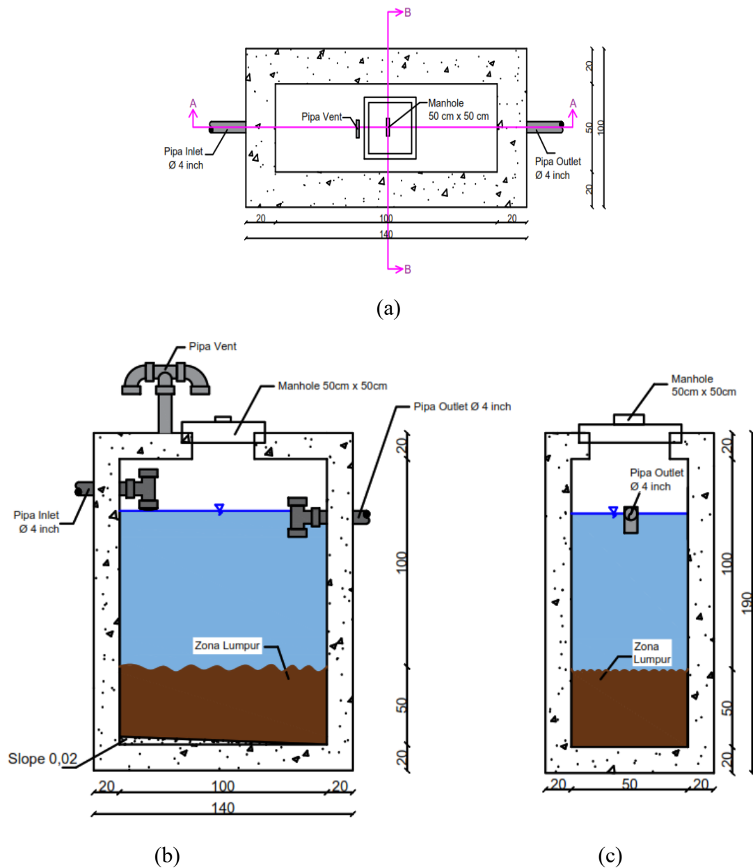
Gambar 9. Desain Unit Pengendap Akhir: (a) tampak atas, (b) potongan A-A, (c) potongan B-B
