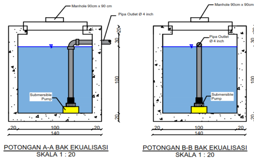
Gambar 5. Desain Bak Ekualisasi : (a) tampak atas, (b) potongan A-A, (c) potongan B-B
