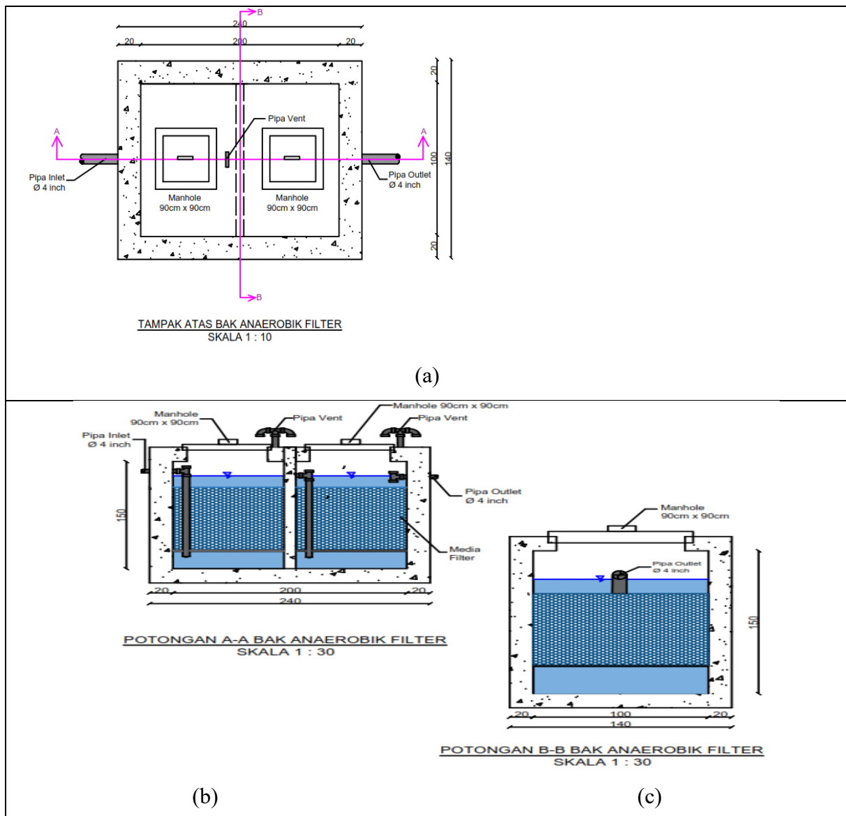
Gambar 7. Desain Unit Anaerobik Filter : (a) tampak atas, (b) potongan A-A, (c) potongan
