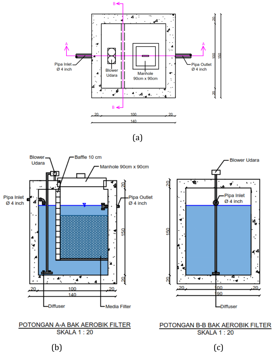
Gambar 8. Desain Unit Aerobik Filter : (a) tampak atas, (b) potongan A-A, (c) potongan B-B
