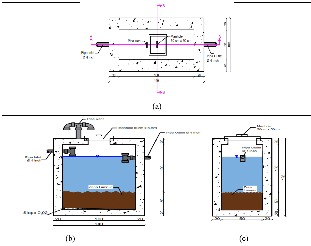
Gambar 6. Desain Unit Pengendap Awal: (a) tampak atas, (b) potongan A-A, (c) potongan B-B
