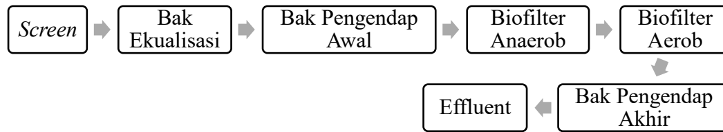
Gambar 3. Diagram Alir Unit Pengolahan
