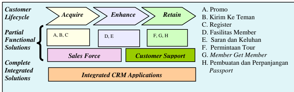
Gambar 2. Arsitektur E-CRM PT. Fajar Buana Internasional
