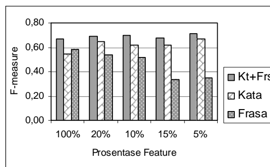
Gambar 3. Rata-rata F-measure pada koleksi T500
