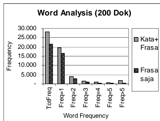
Gambar 2. Frekuensi Kata+Frasa dengan Frasa
