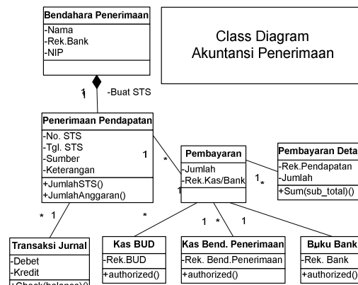
Gambar 2 : Class Diagram akuntansi penerimaan
