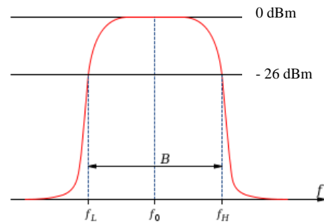
Gambar 1. Karakteristik bandwidth
