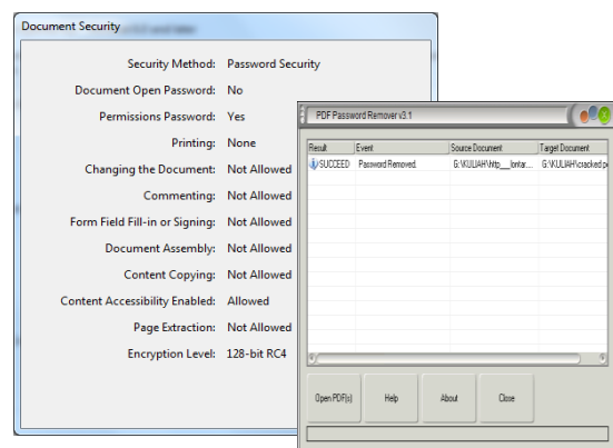
Gambar 1. Parameter Security Dokumen *.pdf
