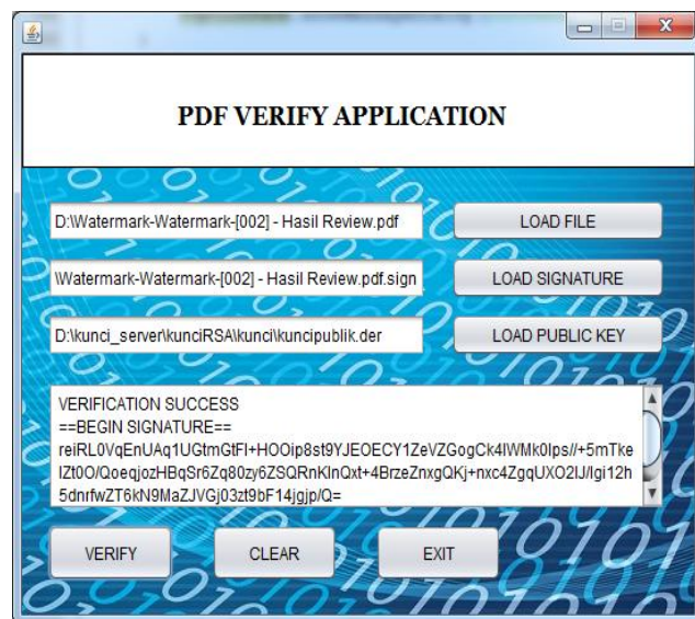
Gambar 13. Implementasi Verifikasi
