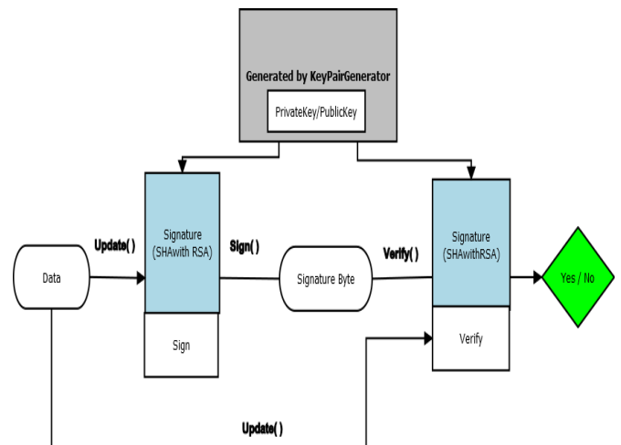
Gambar 9. Proses Signing RSA Memanfaatkan JCE 1
