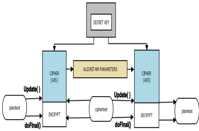
Gambar 10. Proses Enkripsi AES Memanfaatkan JCE 2
