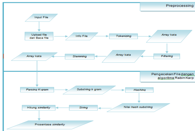
Gambar 3. Arsitektur sistem
