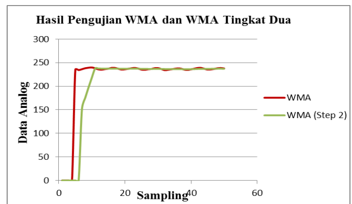
Gambar 5. Hasil Pengujian WMA dan WMA Tingkat Dua
