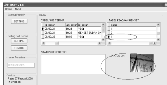
Gambar 5. Tampilan HMI di PC
