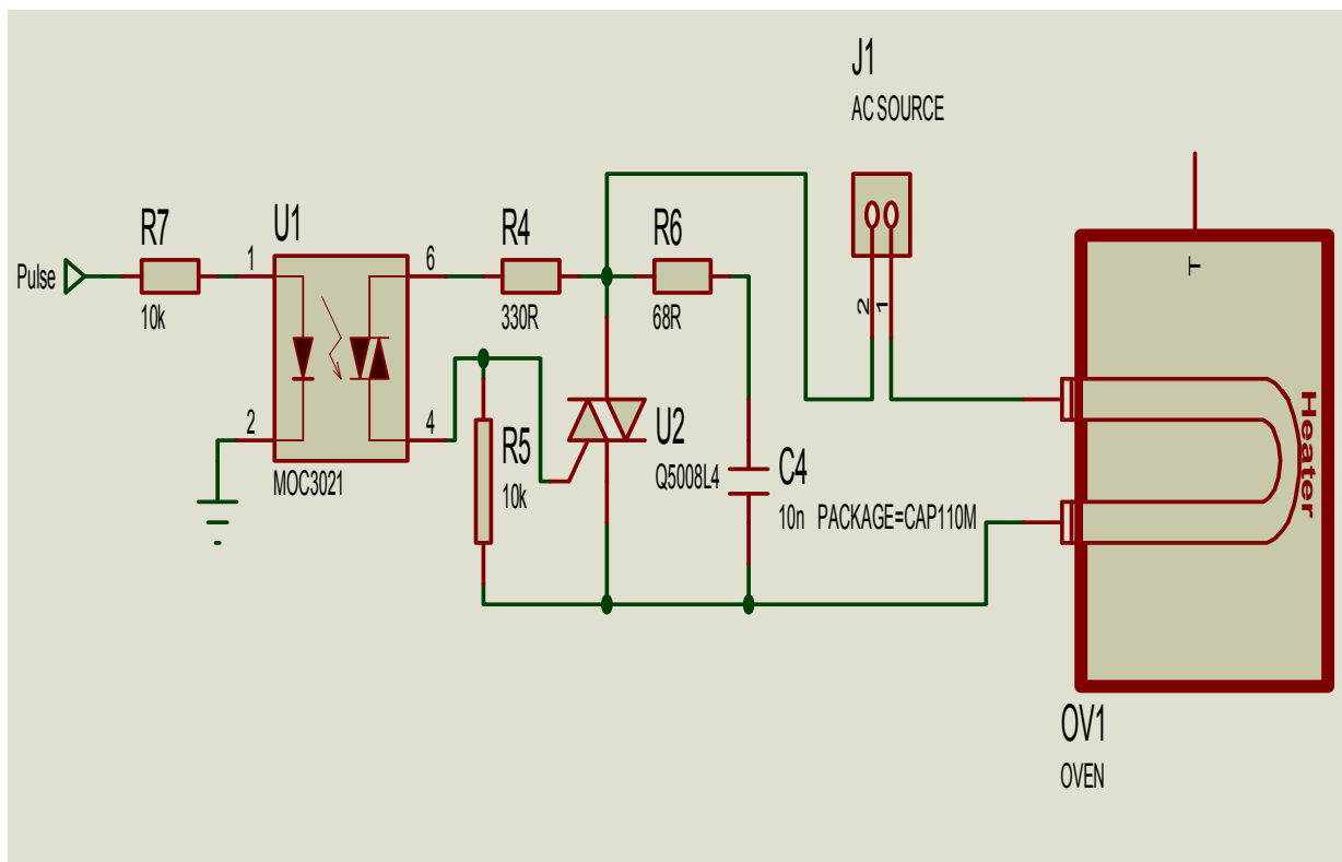
Gambar 12. Rangkaian Heater.
