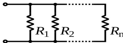
Gambar 7. Hubungan Paralel.
