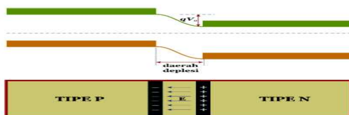
Gambar 4. Diagram Energi Sambungan P-N Munculnya Daerah Deplesi. (Sumber : Ady Iswanto, Staf Divisi Riset 102FM ITB, 2008)
