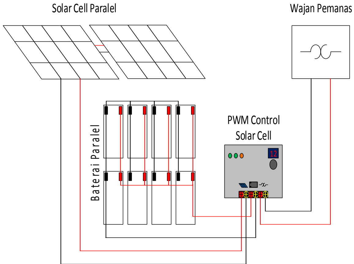
Gambar 13. Gambaran Perancangan Alat.
