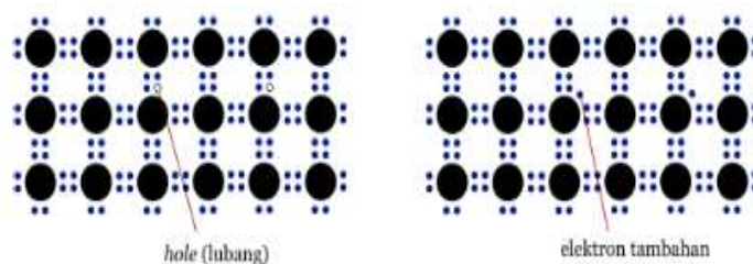
Gambar 3. Semikonduktor Tipe-P (Kiri) dan Tipe-N (Kanan). (Sumber : Ady Iswanto, Staf Divisi Riset 102FM ITB, 2008)
