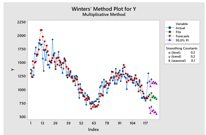
Gambar 8. Analisis Menggunakan Triple Eksponensial Smoothing
