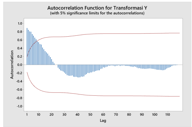
Gambar 5. Plot ACF Data Transformasi
