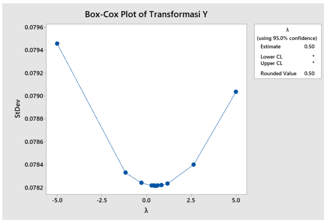
Gambar 4. Box Cox Dari Y Transformasi
