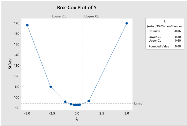
Gambar 3. Box Cox Dari Y
