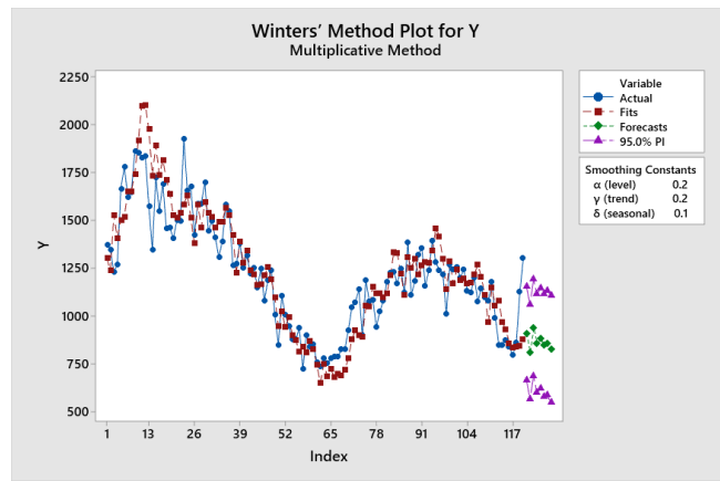
Gambar 9. Peramalan Menggunakan Triple Eksponensial Smoothing
