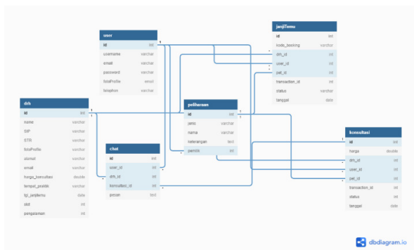
Gambar 6. Tabel Relasi HiVet!.
