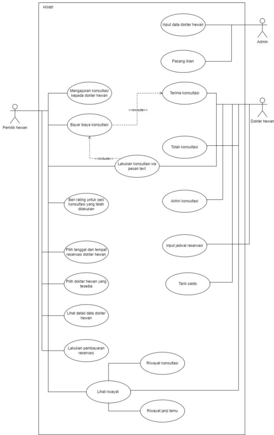
Gambar 5. Use Case Diagram HiVet!.
