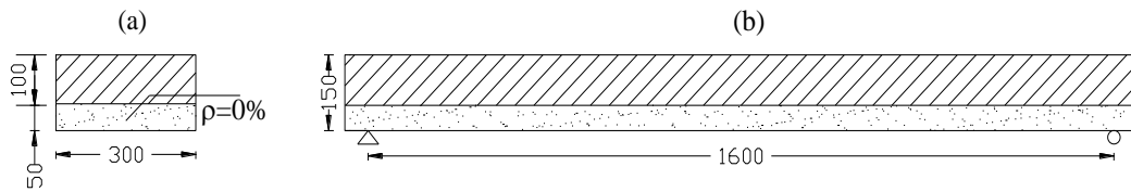
Gambar 5. Penampang melintang (a), memanjang (b) balok B0
